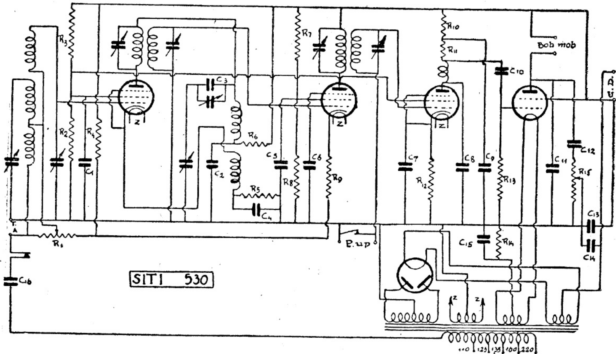
SITI. — Mod. 530. — Valvole: V1 = '57; V2 = '58; V3 = '57; V4 = '47; V5 = '80. — Altri valori non forniti dal Costruttore. — Produzione 1933.
